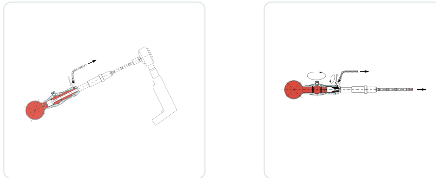
Bild 8: Anbohrgerät nach der Zentrierbohrung (links) bzw. nach der Anbohrung (rechts)
