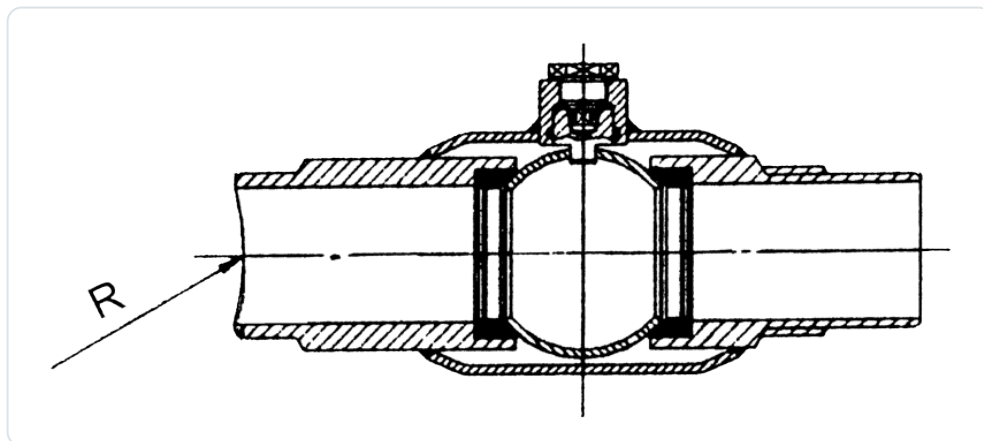
Bild 5: Anpassung der Anschweißendenkontur passend zum Hauptrohr
