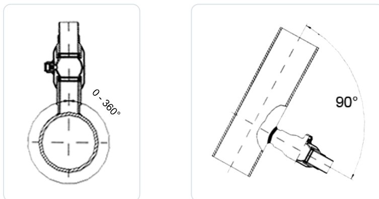
Bild 6: Ausrichtung des Anbohrkugelhahnes zur Rohrleitung
