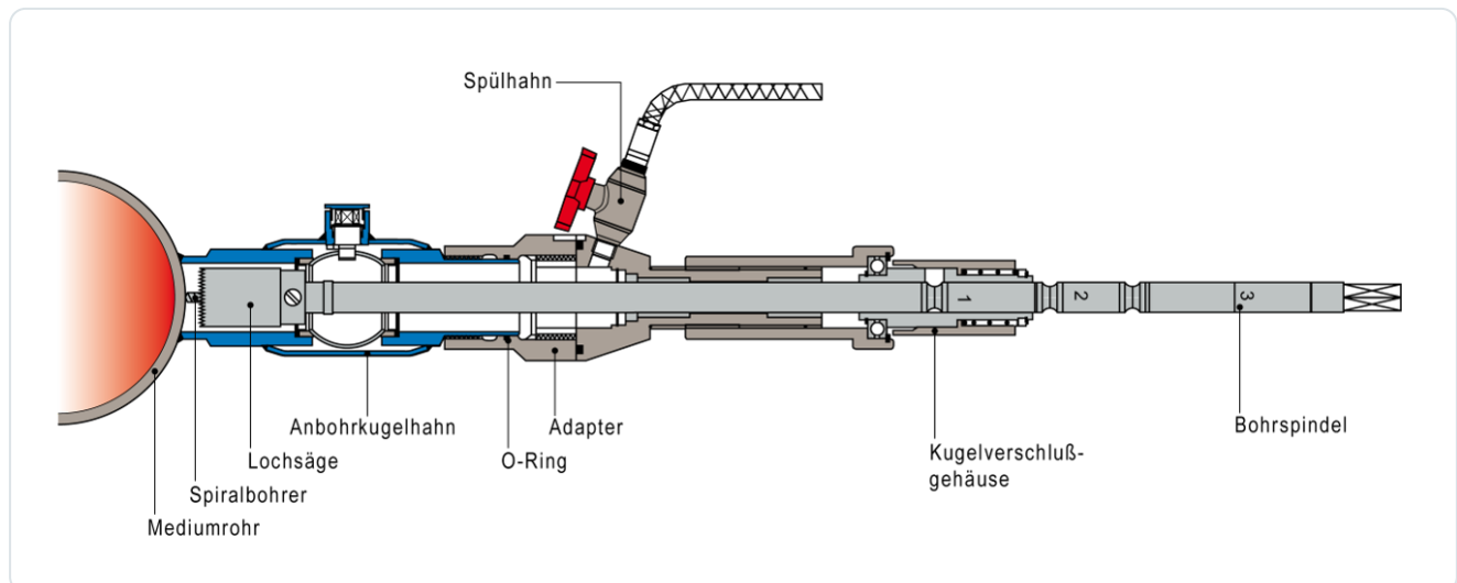
Bild 3: Skizze montiertes Anbohrgerät auf Kugelhahn und Mediumrohr
